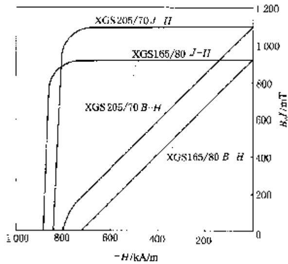
图 B1 XGS 165/80、XGS 205/70 低磁极化强度矫顽力烧结稀土钴永磁材料的典型退磁曲线
