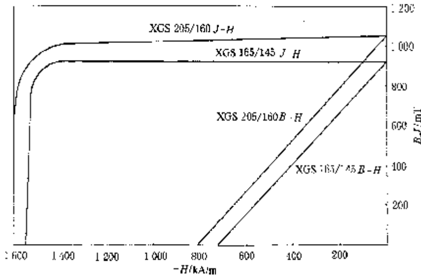
图 B2 XGS 165/145、XGS 205/160 高磁极化强度矫顽力烧结稀土钴永磁材料的典型退磁曲线
