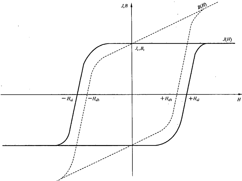
图 1 磁滞回线
